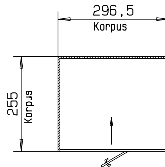
Grundriss
