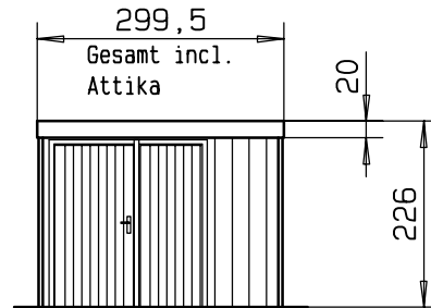
Vorderansicht
