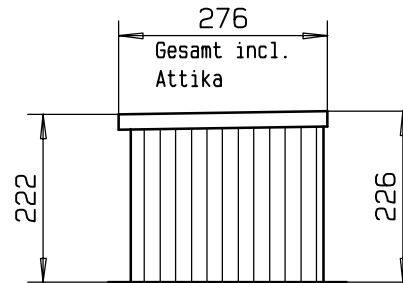
Seitenansicht, links
