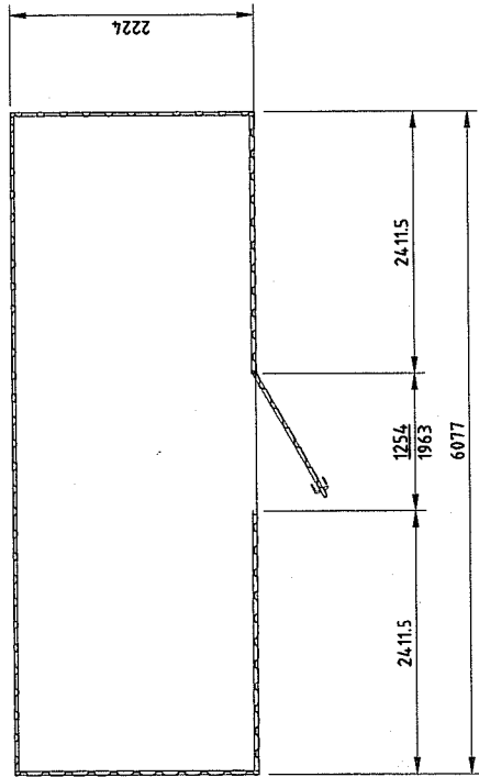
GRUNDRISS
