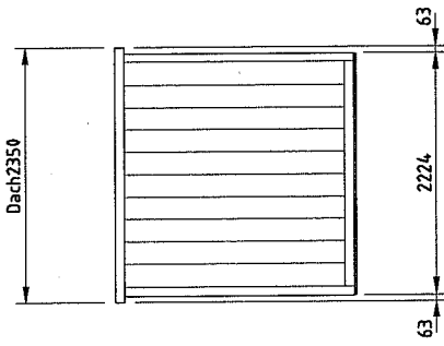
SEITENWAND
