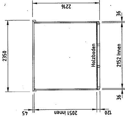
QUERSCHNITT
