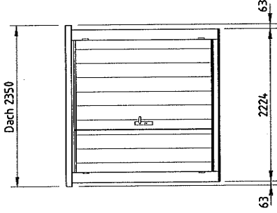
SEITENWAND
