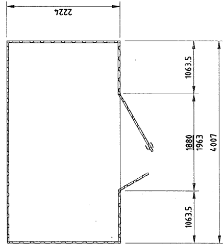
GRUNDRISS
