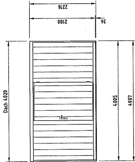
TÜR/WAND
