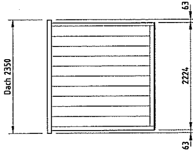
SEITENWAND
