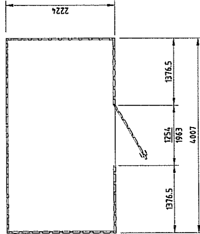
GRUNDRISS
